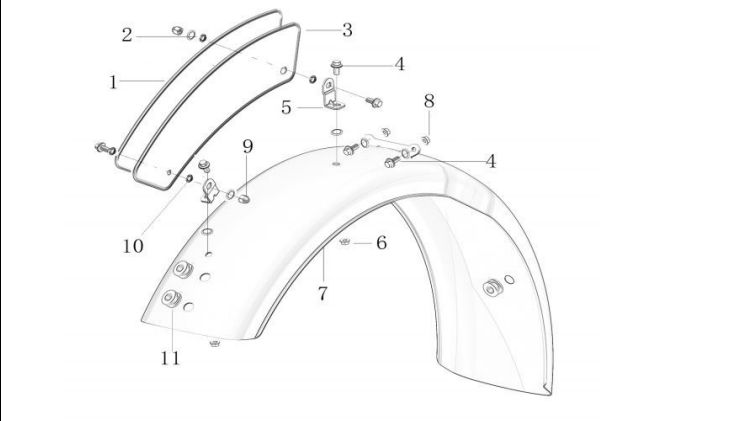
F-15 前挡泥板/FRONT FENDER
