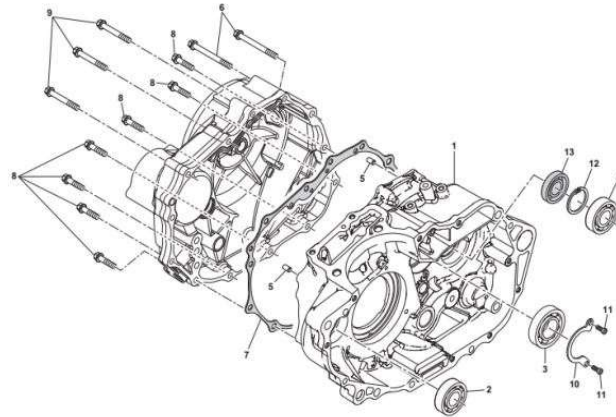
E-9 右曲轴箱 R-CRANKCASE
