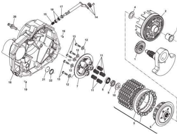
E-10 离合器CLUTCH
