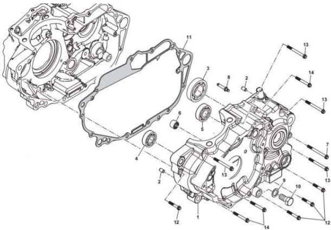
E-8 左曲轴箱 L-CRANKCASE
