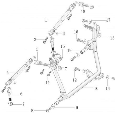
F-21 边车连接部分/ JOINT PART
