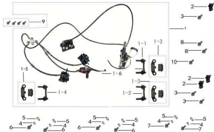
前制动总成
