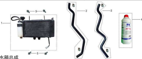
水箱总成
