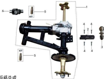
后桥总成
